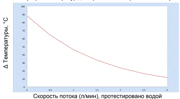
График температур для проточного нагревателя материала
