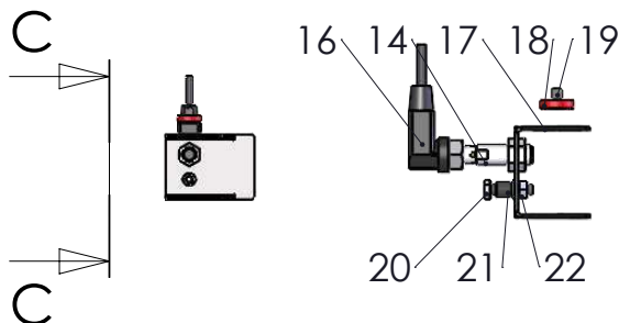
SCHNITT C-C MABSTAB 1 : 5
