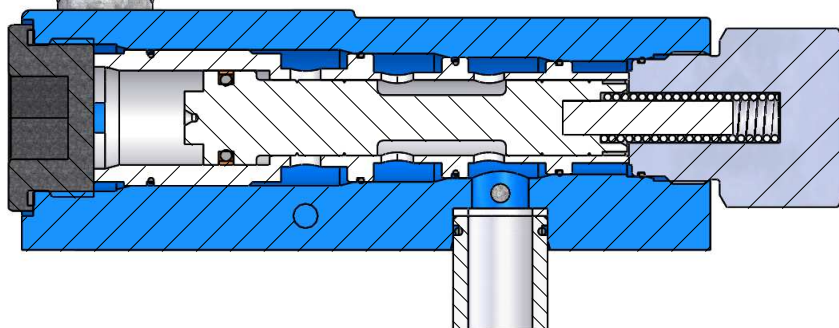
SCHNITT C-C MAßSTAB 1 : 2
