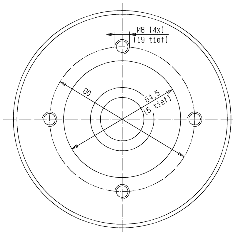
Ansicht A (Pos.43)
