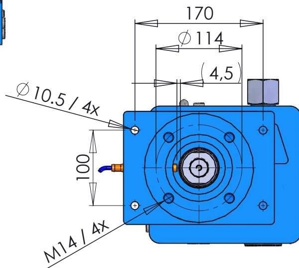
ANSICHT B
