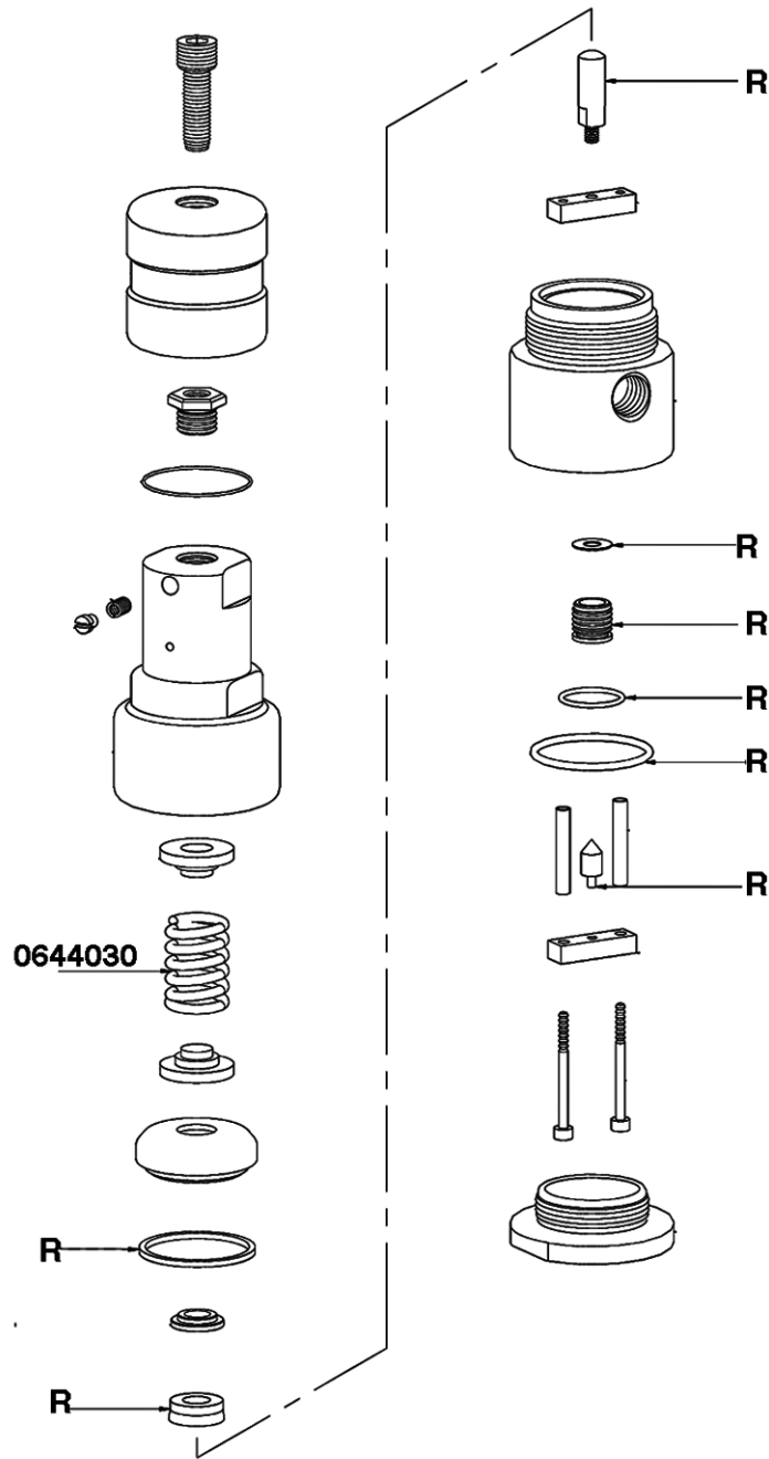
R=Reparaturset=repair kit=jeu de réparation 0644434
