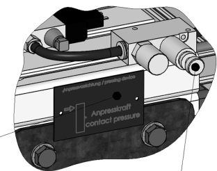
Ansicht B
