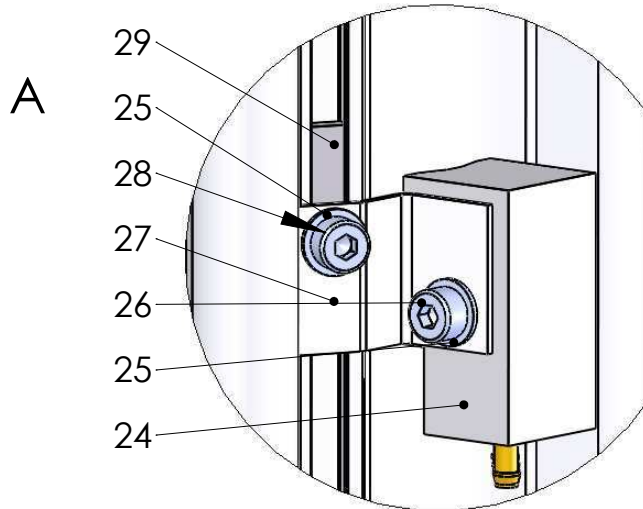
DETAIL A Maßstab 1 : 1
