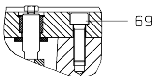
Schnitt A-B
