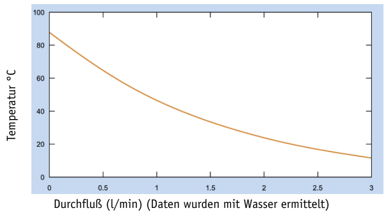
Temperaturschaubild Materialdurchflußerhitzer
